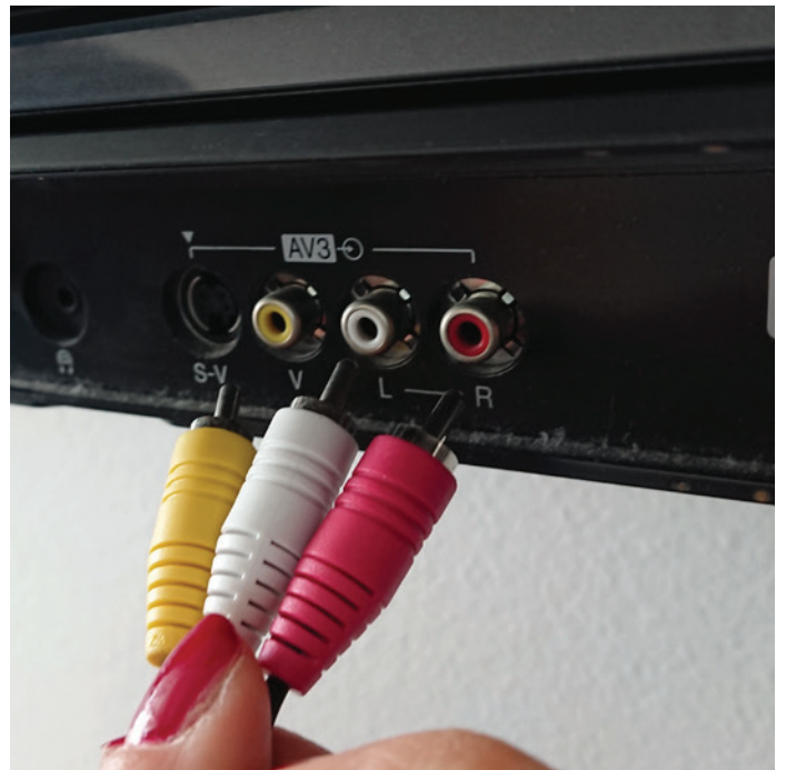
Drugo stran SCART kabla vključite v tako pripravljen vhod na TV sprejemniku.
